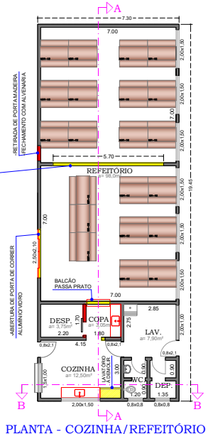
PLANTA - COZINHA/REFEITÓRIO
